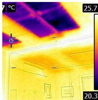
Ejemplo de funcionamiento en modo refrescamiento
