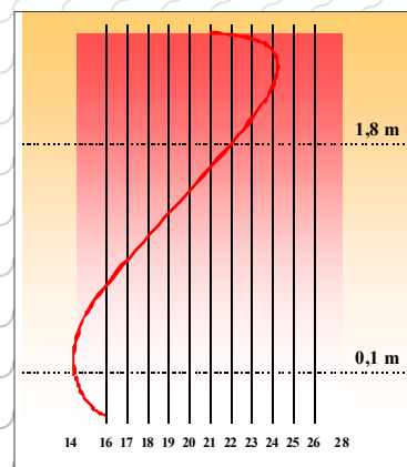
Calefacción tradicional por radiadores
