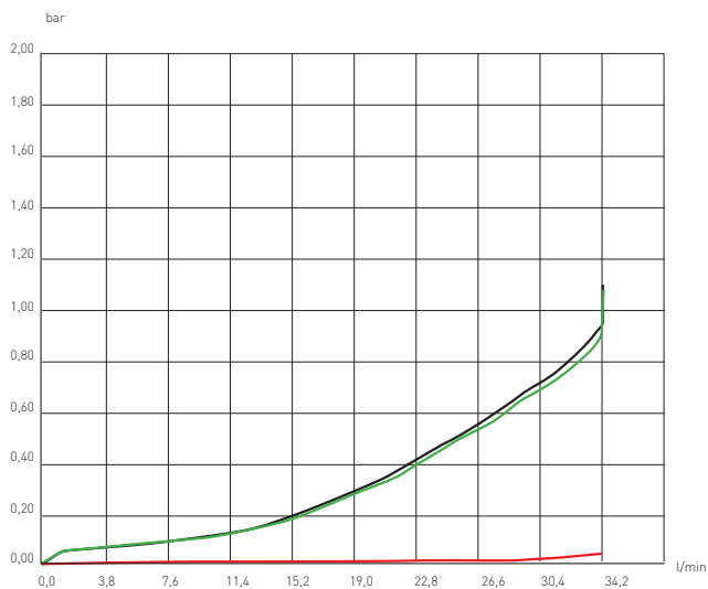
MÓDULO DE IDA CON CAUDALÍMETRO
